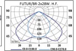
LOR = 45.31%
